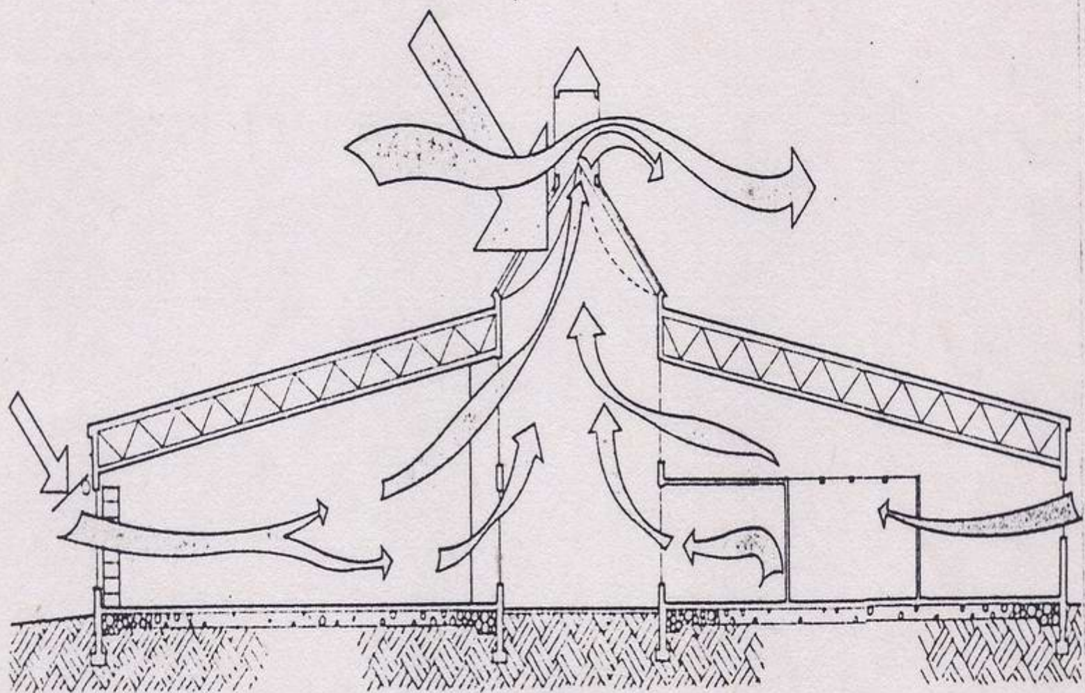
自然通風系統 利用上升氣流及風壓誘導通風
